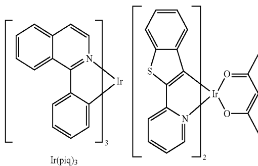
Btp 2 Ir(acac)
